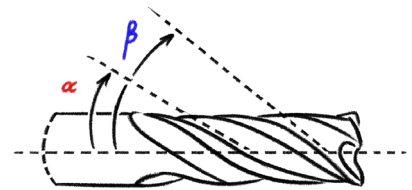
Unterschiedlicher Drallwinkel
