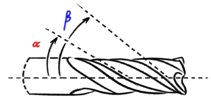
Unterschiedlicher Drallwinkel
